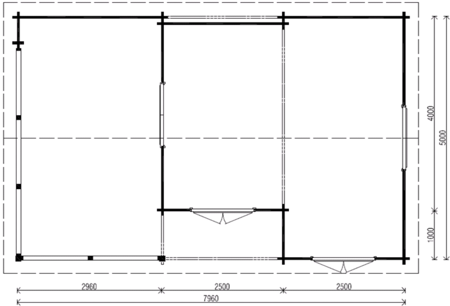
Plattegrond JR 20035
