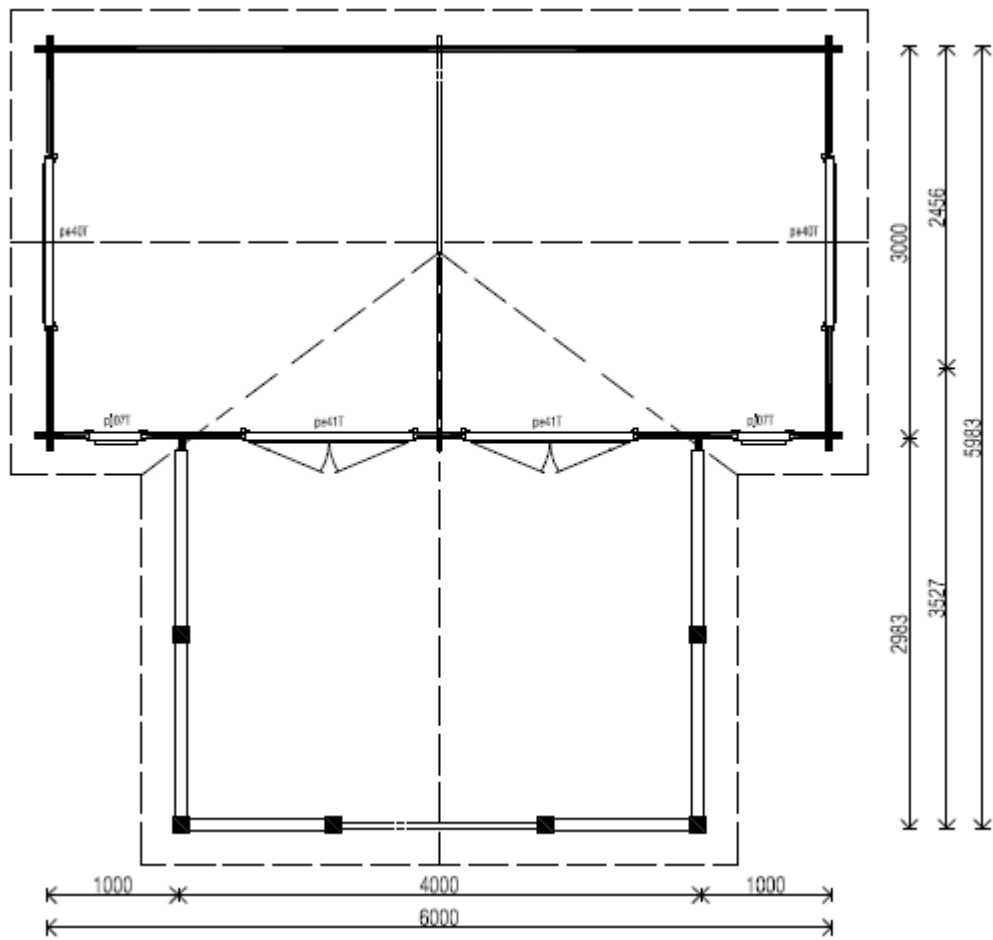
Plattegrond
