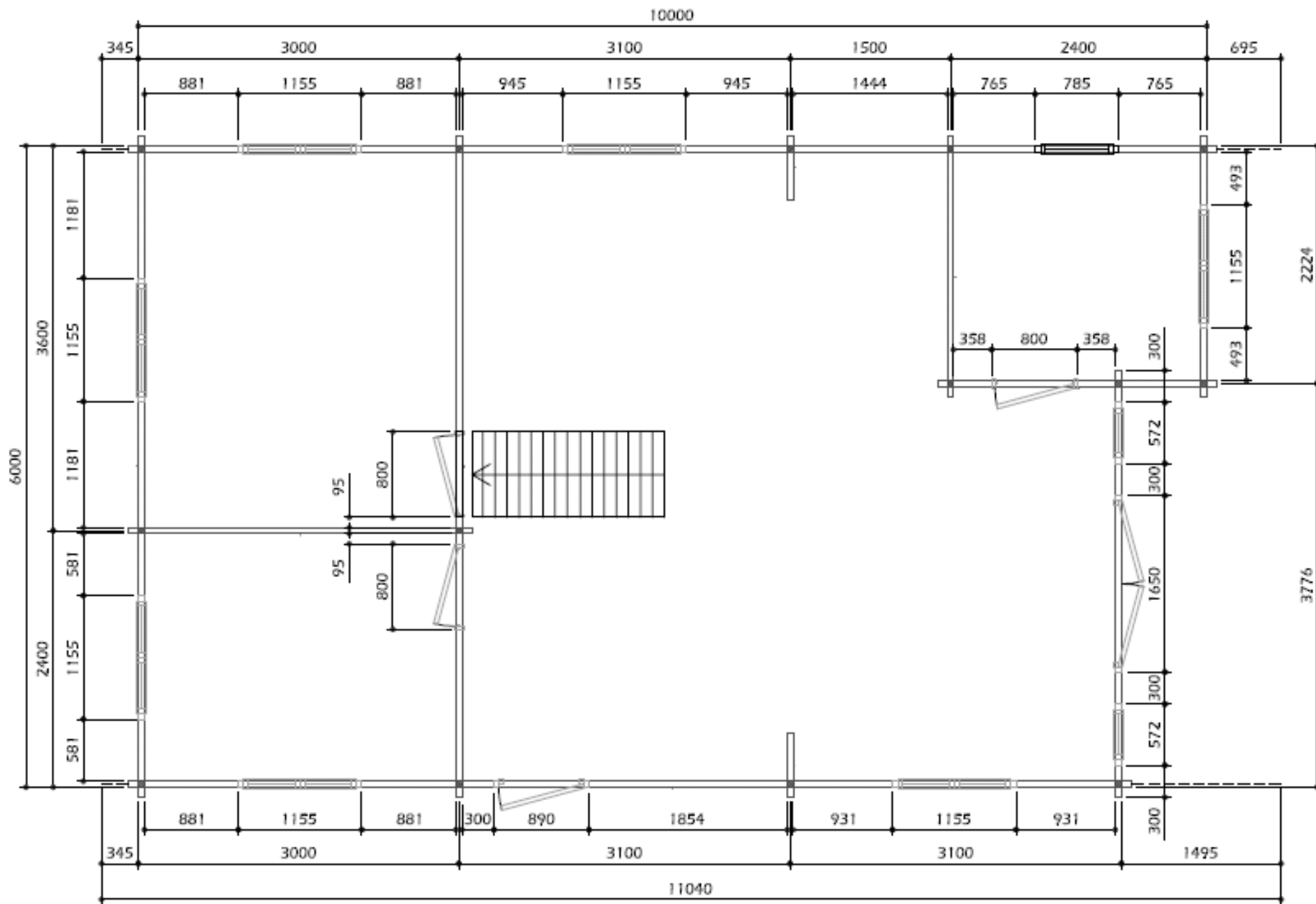
Grondplan JR 20040 gelijkvloers
