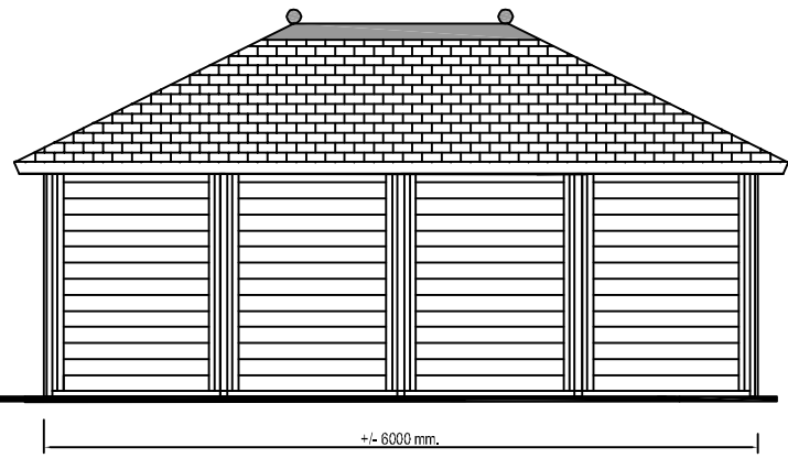
Achter aanzicht Hinten Ansicht Rear view
