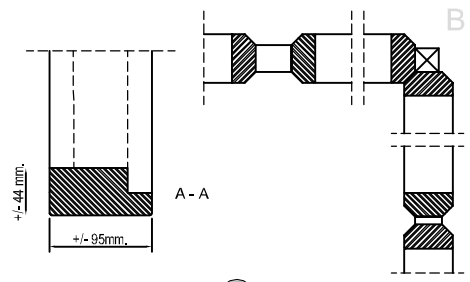
Achter aanzicht Hinten Ansicht Rear view
